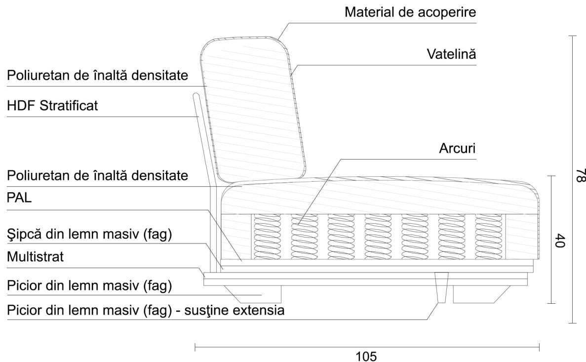
Canapea 3L Ext B Mare
